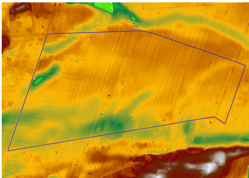
Mapa 3 Hipsometria obszaru opracowania
