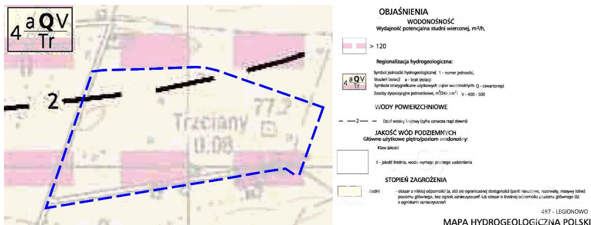
Mapa 9 - Obszar opracowania w kontekście fragmentu mapy hydrogeologicznej - arkusz Legionowo
