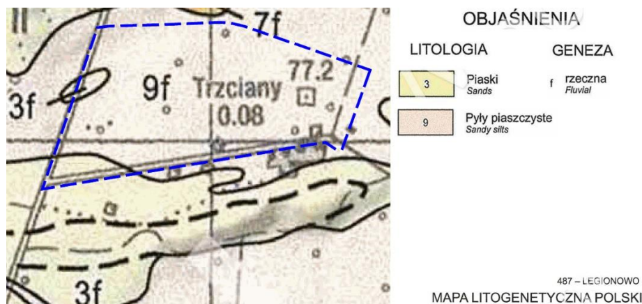
Mapa 4 Obszar opracowania w kontekście fragmentu mapy litogenicznej – arkusz Legionowo
