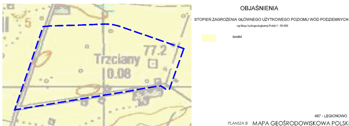
Mapa 10 Obszar opracowania w kontekście fragmentu mapy geośrodowiskowej plansza B - arkusz Legionowo
