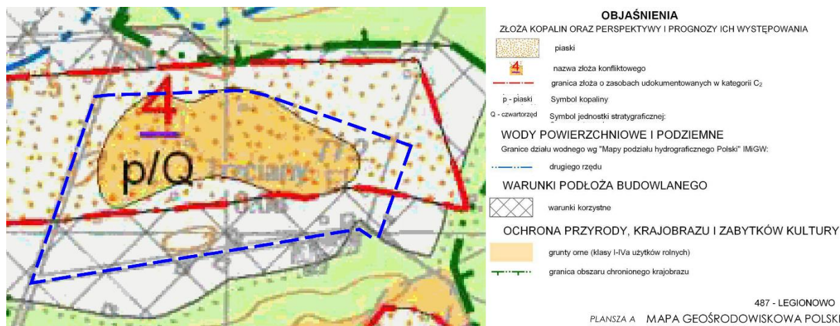
Mapa 13 - Obszar opracowania w kontekście fragmentu mapy geologicznej – arkusz 487
