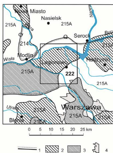
Fig. 3. Położenie arkusza Legionowo na tle obszarów głównych zbiorników wód podziemnych (GZWP) w Polsce wymagających szczególnej ochrony, w skali 1:500 000 wg A. S. Kieczkowskiego, red. (1990)
