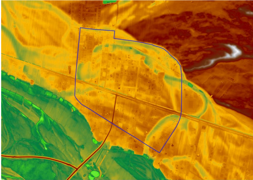
Mapa 3 Hipsometria obszaru opracowania
