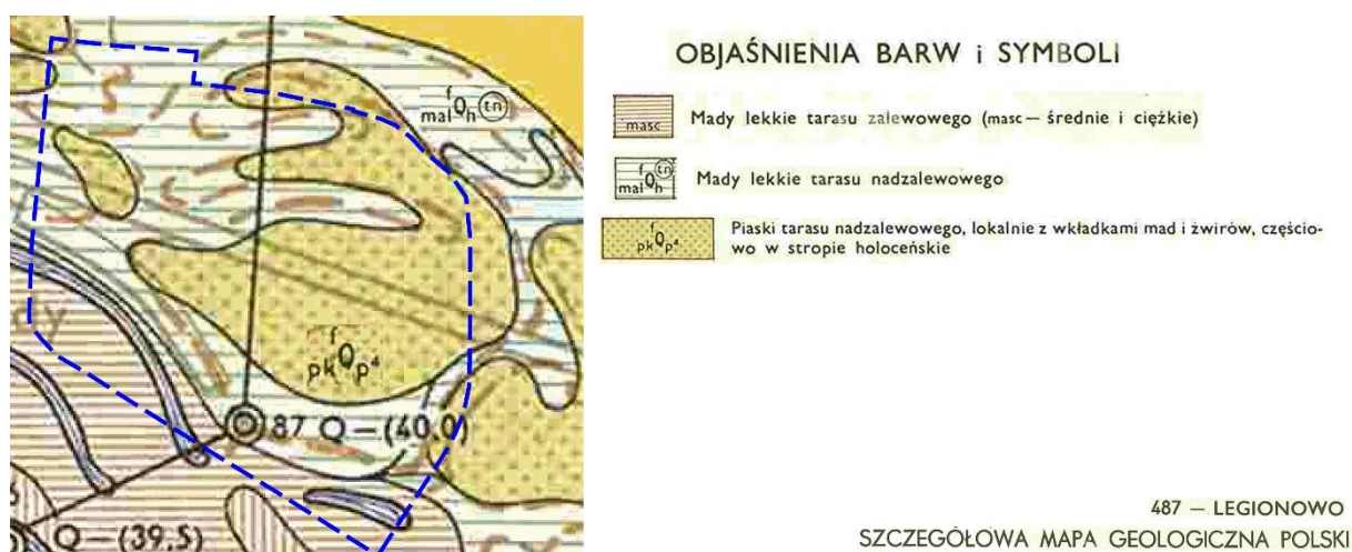
Mapa 5 – Obszar opracowania w kontekście fragmentu Szczegółowej Mapy Geologicznej Polski, arkusz Legionowo
