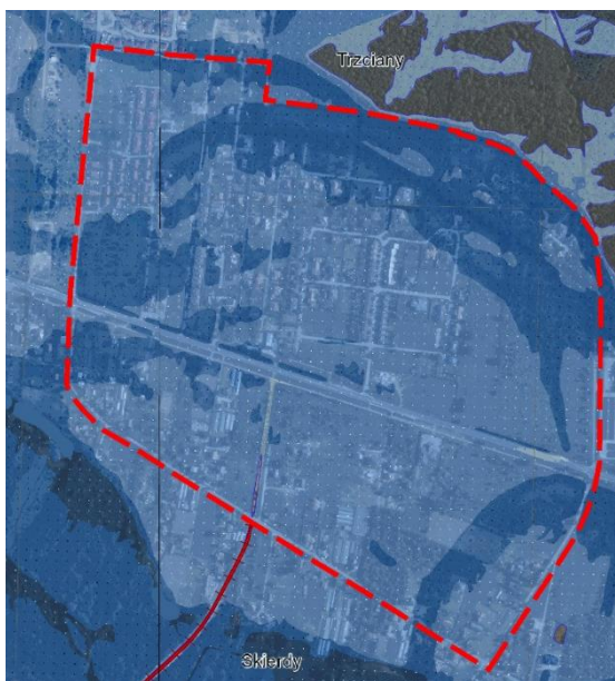
Mapa 10 Mapa zagrożenia powodziowego wraz z głębokością wody. Obszary narażone na zalanie w przypadku zniszczenia lub uszkodzenia wału przeciwpowodziowego
