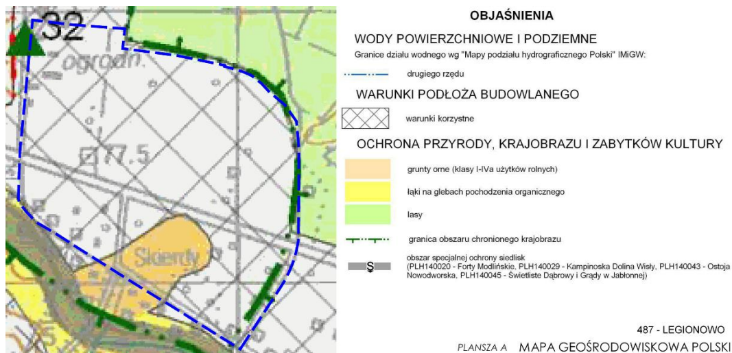
Mapa 12 - Obszar opracowania w kontekście fragmentu mapy geologicznej – arkusz 487
