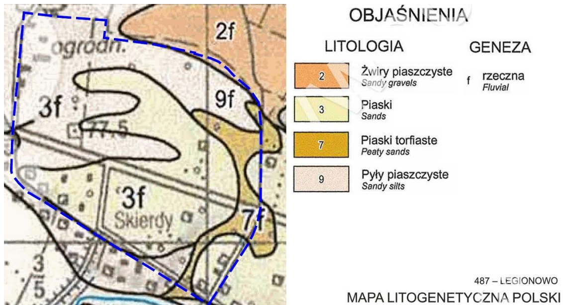
Mapa 4 Obszar opracowania w kontekście fragmentu mapy litogenicznej – arkusz Legionowo
