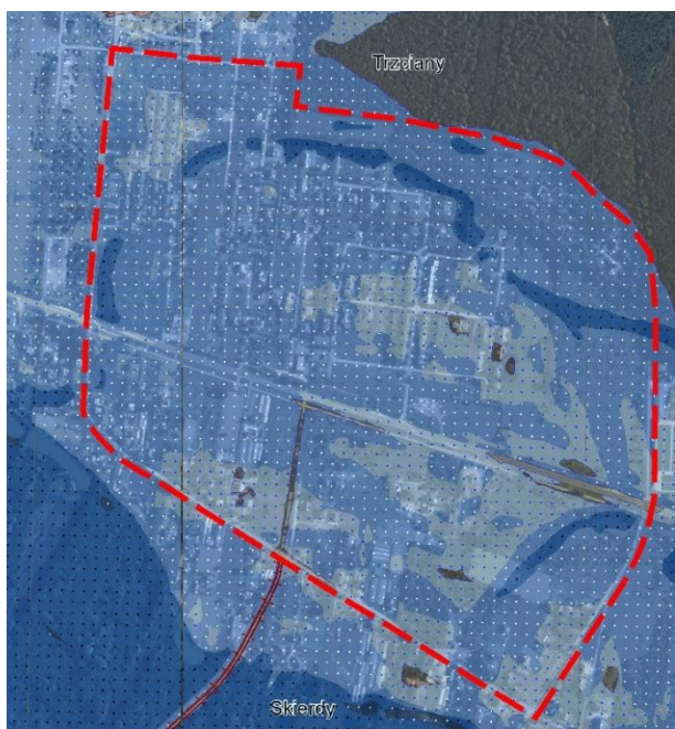
Mapa 11 Mapa zagrożenia powodziowego terenów na których prawdopodobieństwo wystąpienia powodzi jest niskie i wynosi raz na 500 lat lub na którym istnieje prawdopodobieństwo wystąpienia zdarzenia ekstremalnego
