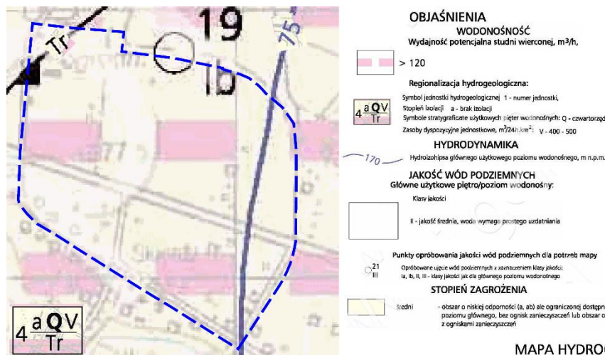
Mapa 8 - Obszar opracowania w kontekście fragmentu mapy hydrogeologicznej - arkusz Legionowo
